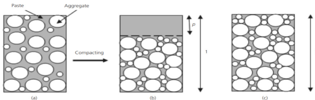
Рисунок 1: Иллюстрация частиц для расчета средней толщины цементной пасты: (а) бетонная смесь; (б) сжатый бетон; (с) сжатый бетон
