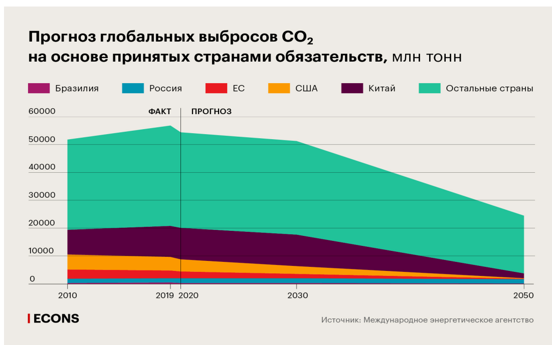
Рис.1 Прогноз глобальных выбросов CO 2 .
