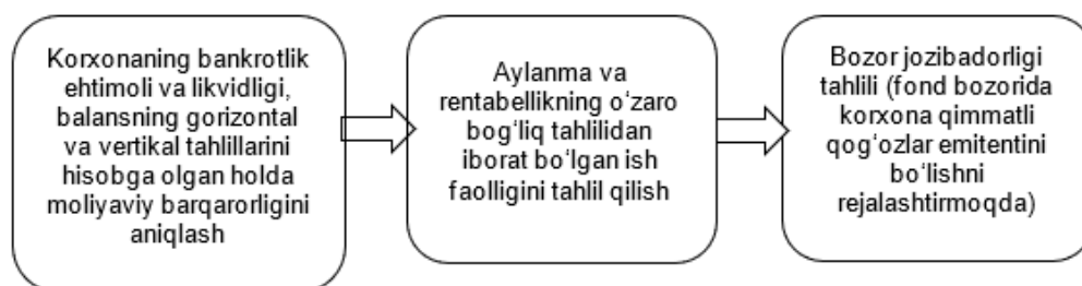
2-rasm: Korxona moliyaviy barqarorligini tahlil qilishning neoklassik chizmasi [10]
