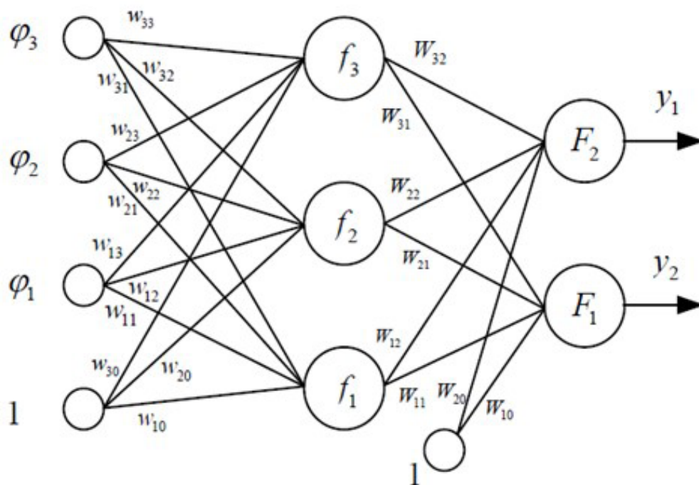
1-rasm: Ikki qatlamli neyron tarmog'ining ko'rinishi
