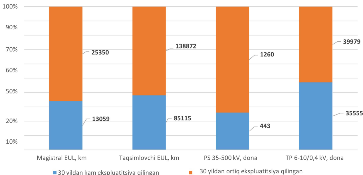
3-rasm: Elektr tarmoqlarining holati 6
