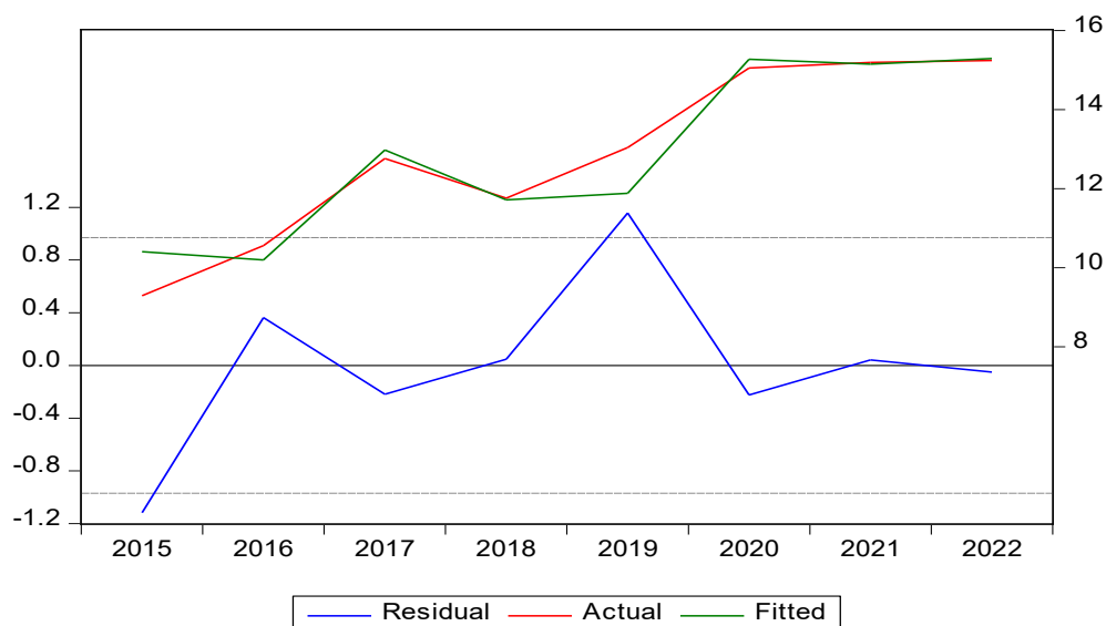
1-rasm: "O'zneftgaz" aksiyadorlik kompaniyasi korxonalari tomonidan olingan sof foyda (zarar) hajmining qoldiq, haqiqiy va tuzilgan model qiymatlari grafigi 3
