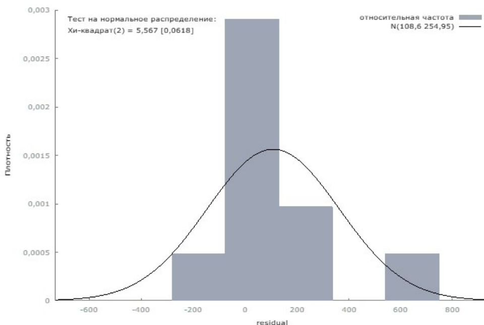
4-rasm: Model qoldiqlarining ehtimollilik ko'rsatkichi 8
