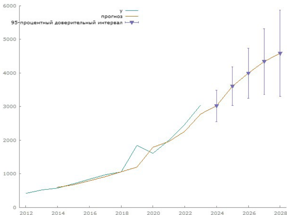
5-rasm: Vaqtli qatorning tekislangan va haqiqiy darajalari hamda prognoz qiymatlari 9
