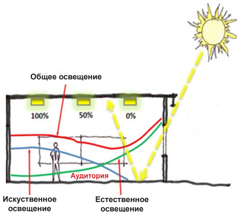
Рис. 2: Комбинированное освещение
