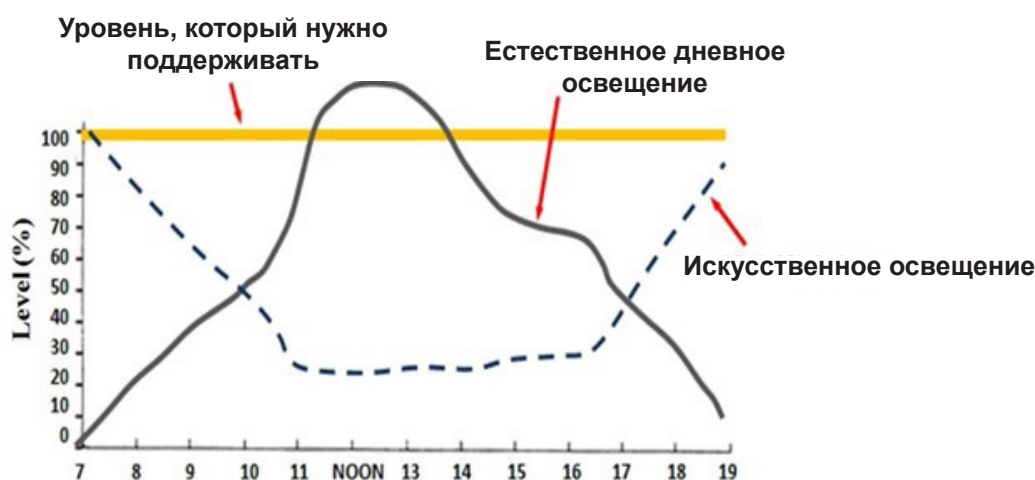
Рис.1: Принципы стратегии комбинированного освещения: повышение уровня освещенности за счет использования искусственного освещения в местах, где естественного освещения недостаточно
