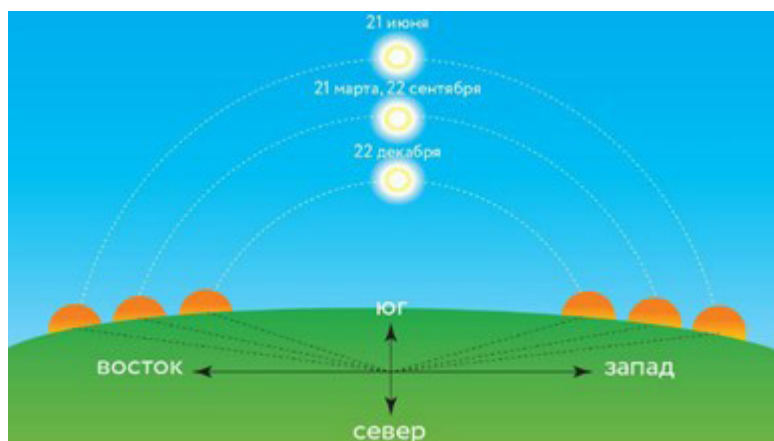
Рис. 5: Видимое движение солнца.
