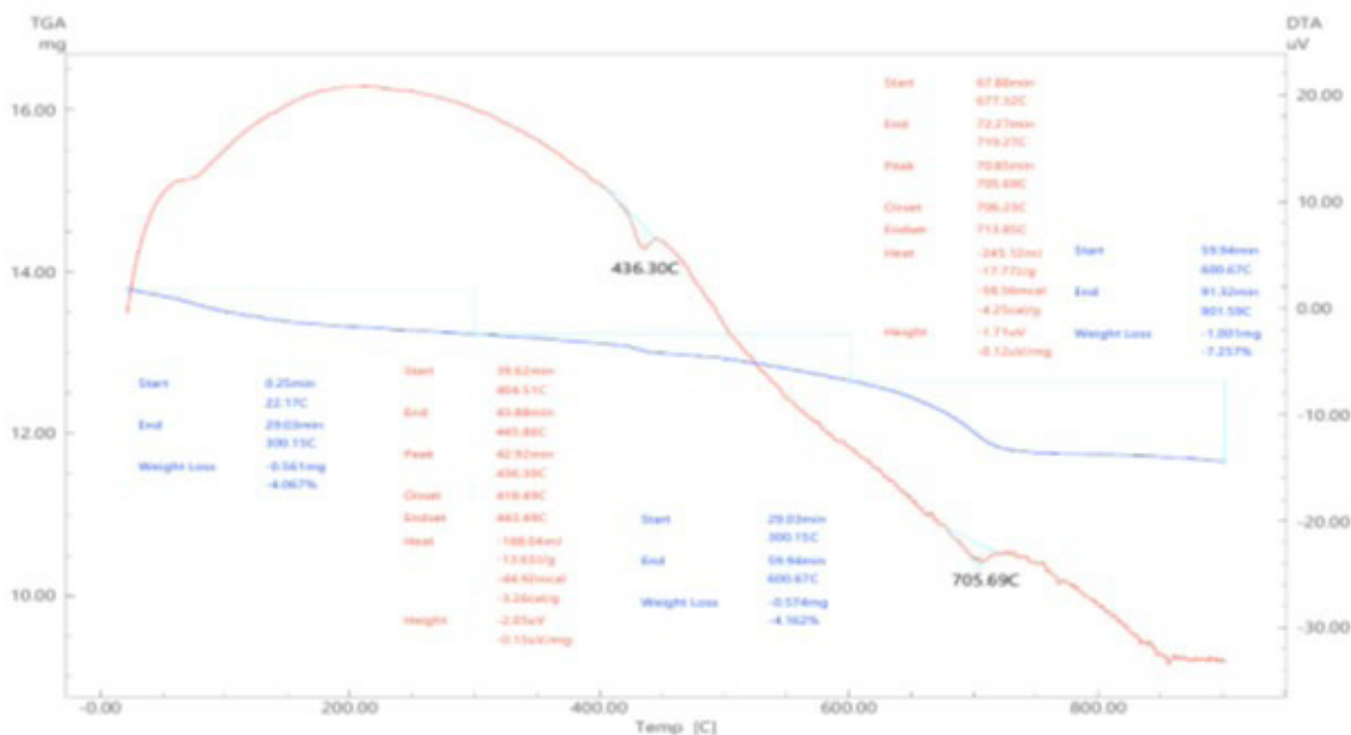
2-rasm: S-1 superplastifikator qo'shimchasining 0,8% qo'shilgan betonni termik tahlili
